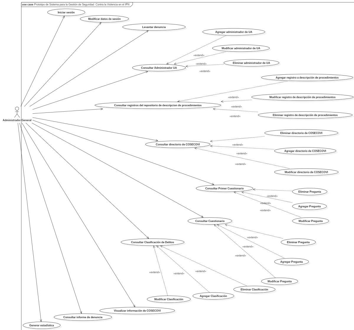
Figura 11 Casos de Uso de Administrador General
