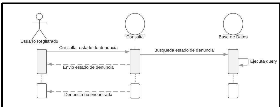
Figura 31 Diagrama de secuencia consultar estado de la denuncia.
