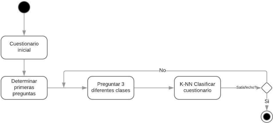
Figura 85 Diagrama de funcionamiento K-NN.
